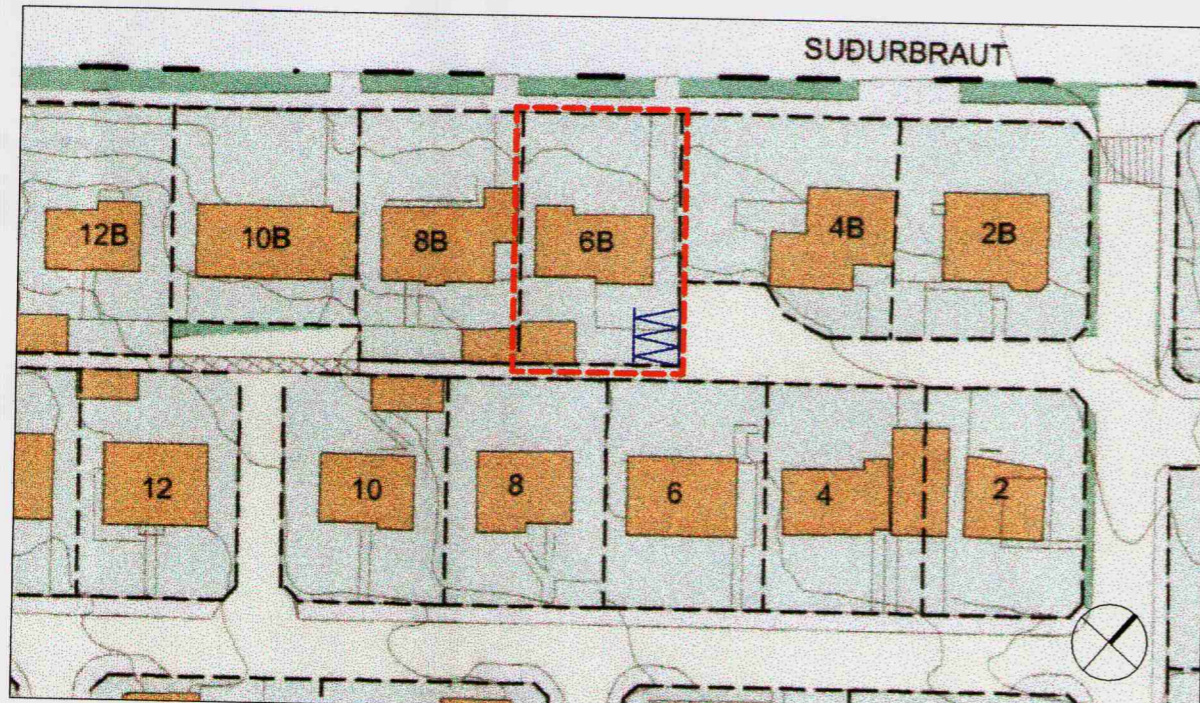
DEILISKIPULAG EFTIR BREYTINGU MKV. 1:1000
