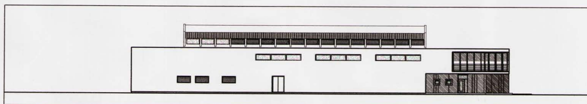
ÚTLIT NORÐUR EFTIR BREYTINGAR
