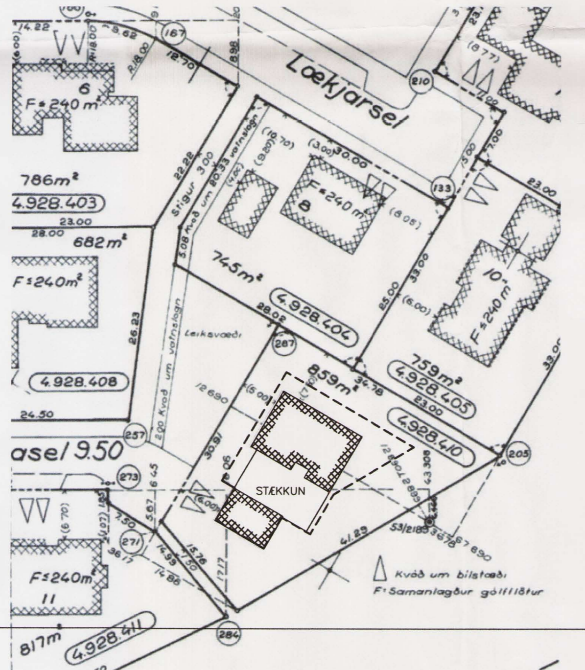
TILLAGA AÐ BREYTTU MÆLIBLADI, SEM SÝNIR STÆKKUN HÚSS. SKÝRINGARMYND, M. 1:500
