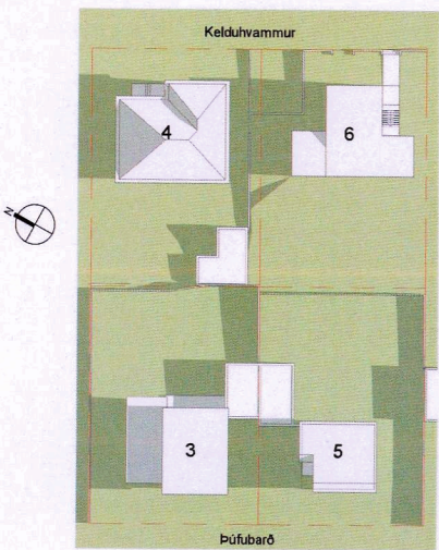
vorjafndægur kl 12
