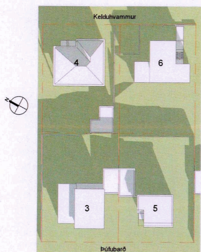
vorjafndægur kl 16
