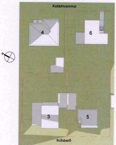
vetrarsólstöður kl. 12
