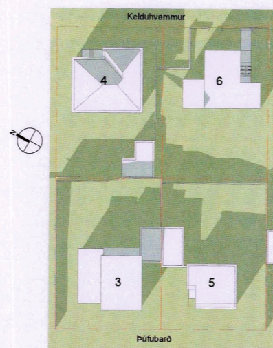
sumarsólstöður kl. 19
