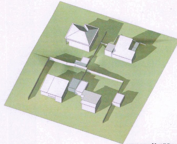
sumarsólstöður kl. 19
