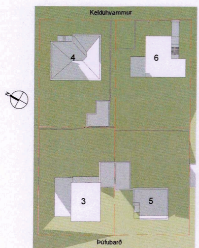
vetrarsólstöður kl. 16
