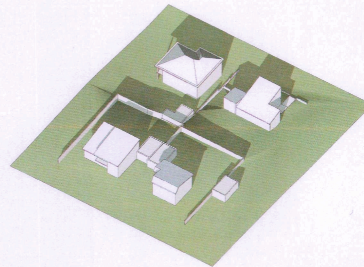
vorjafndægur kl. 16
