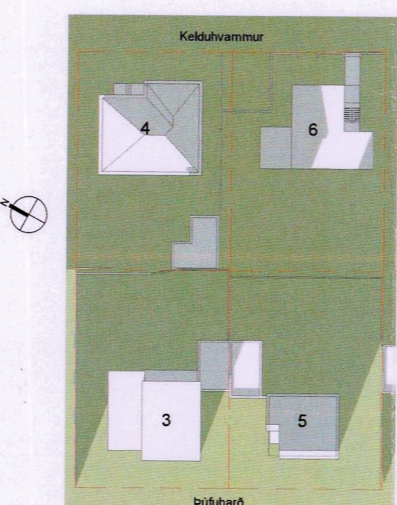
vorjafndægur kl 19
