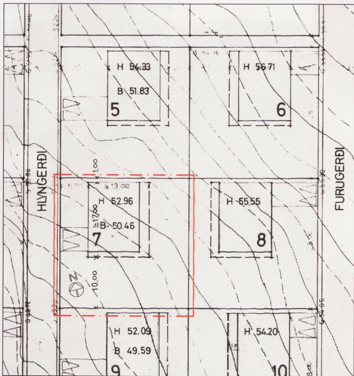
HLUTI GILDANDI DEILISKIPULAGS "ESPIGERÐI" SAMÞYKKT Í BORGARRÁÐI 3. 11. 1971 M-1:500
