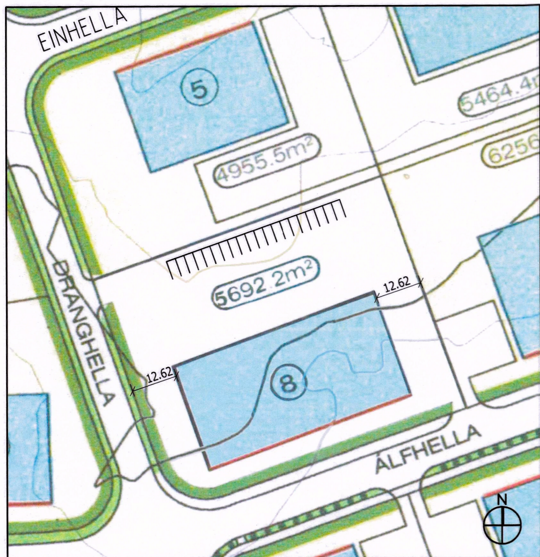
GILDANDI DEILISKIPULAG HELLNAHRAUN 2. áfangi MKV 1:1000 SAMÞYKKT 15.05.2007 MEÐ SÍÐARI BREYTINGUM.
