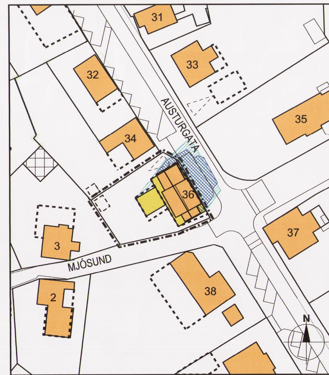
Sumarsólstöður kl. 16:00
