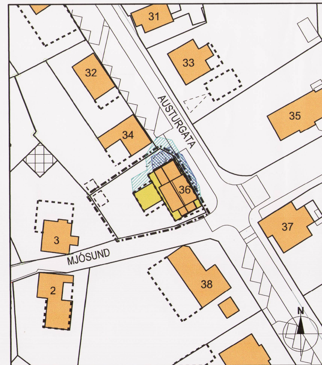
Sumarsólstöður kl. 13:00
