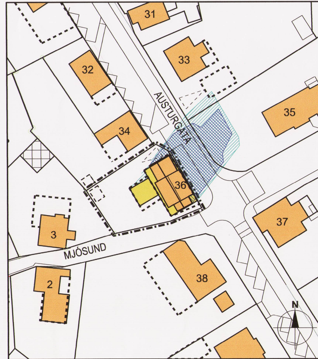
Jafndægur kl. 16:00
