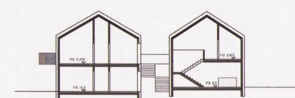
Snið C-C
