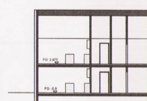
Snið B-B
