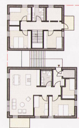
Grunnmynd 2. hæð
