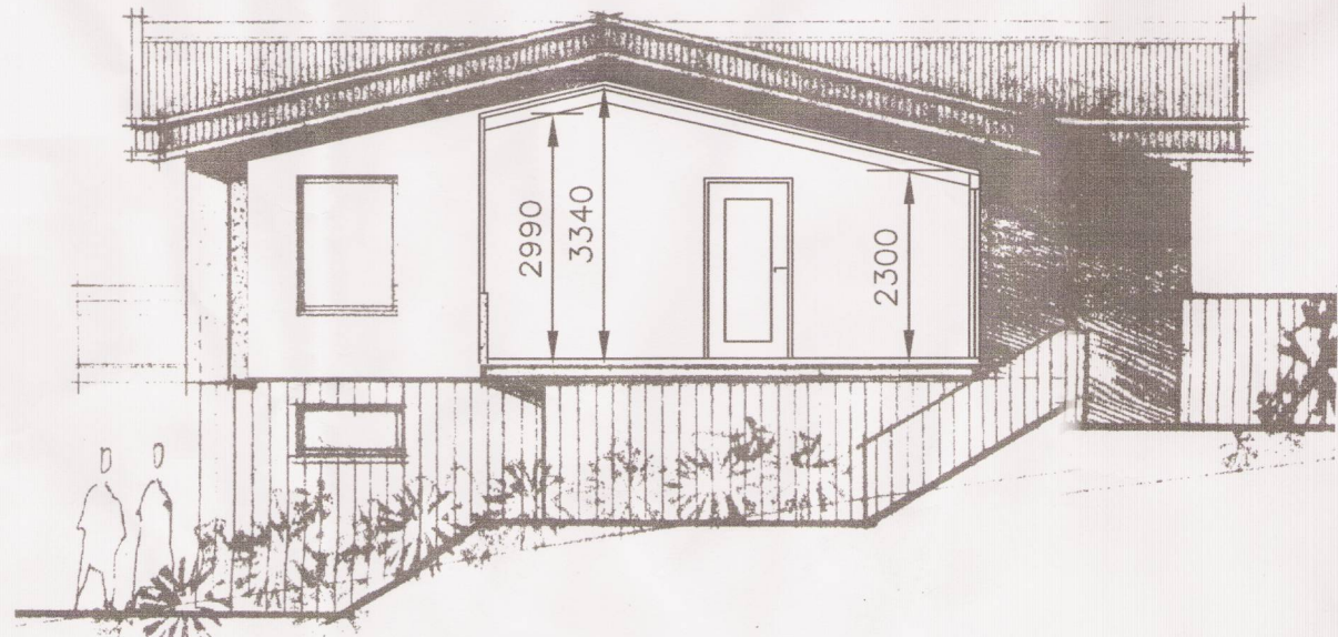
SKÝRINGARTEIKNING, SNIÐ. 1:100
