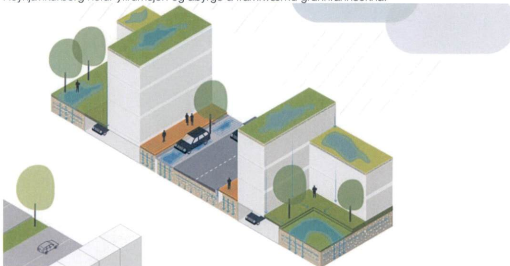
Myndin sýnir meginreglu fyrir ofanvatnslausnir
