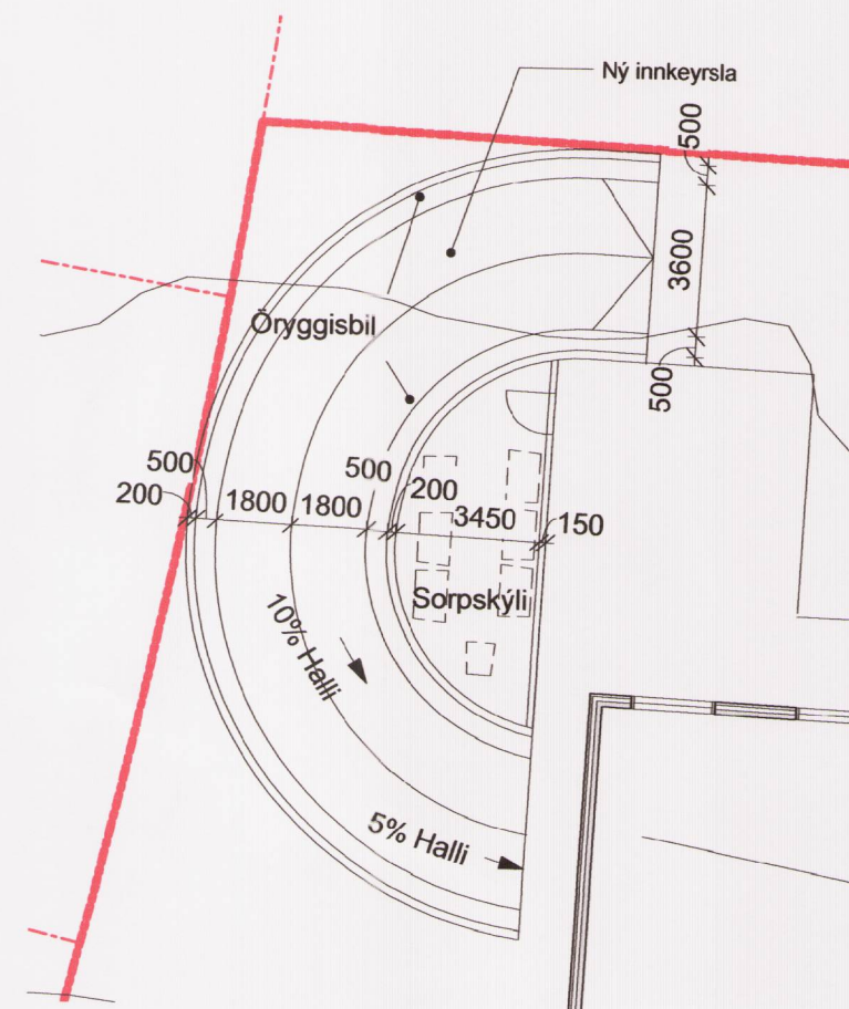
2 Skýringarmynd, skábraut 1 : 200
