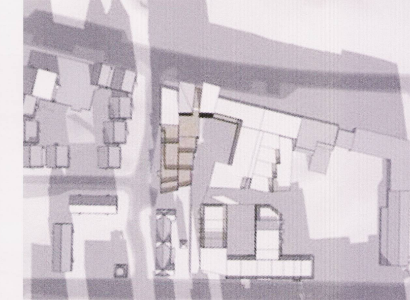
JAFNDÆGUR KL 13:30
