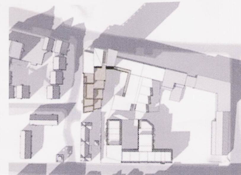
SUMARSÓLSTÖÐUR KL 16:00
