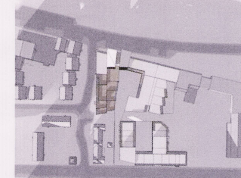
JAFNDÆGUR KL 16:00
