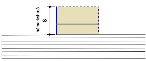
E3 fjölbýli, skilmálateikning - kvöð
