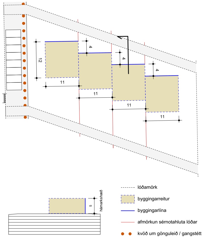
C keðjuhús, skilmálateikning
