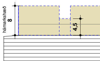
D2 fjölbýli - sérhæðir, skilmálateikning
