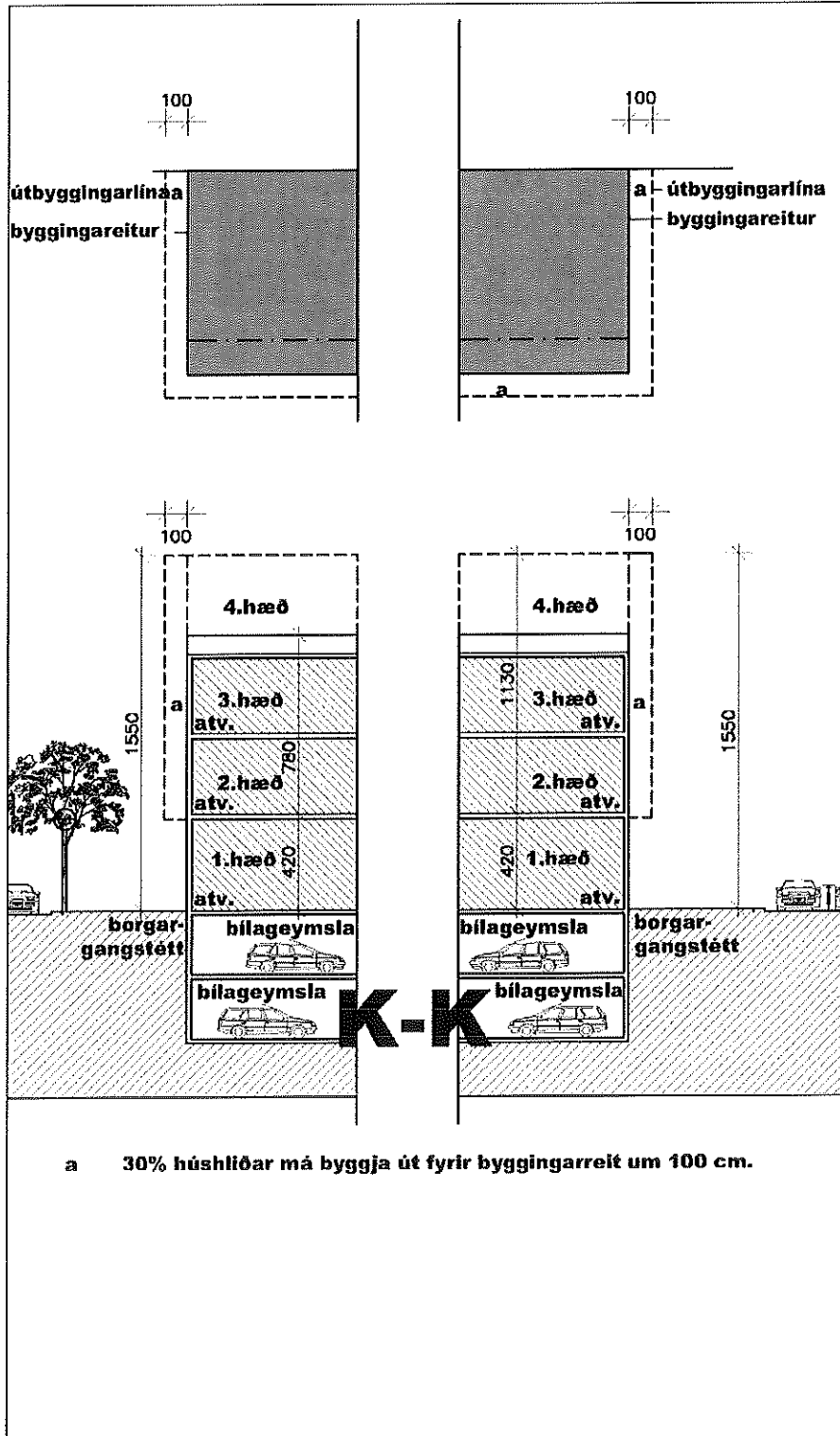
Skilmálasnið K-K
