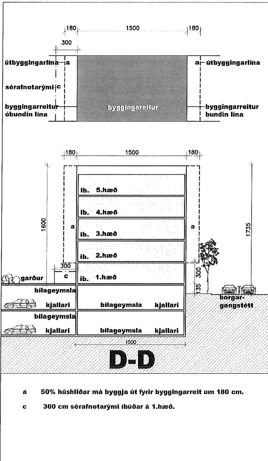
Skilmálasnið D-D
