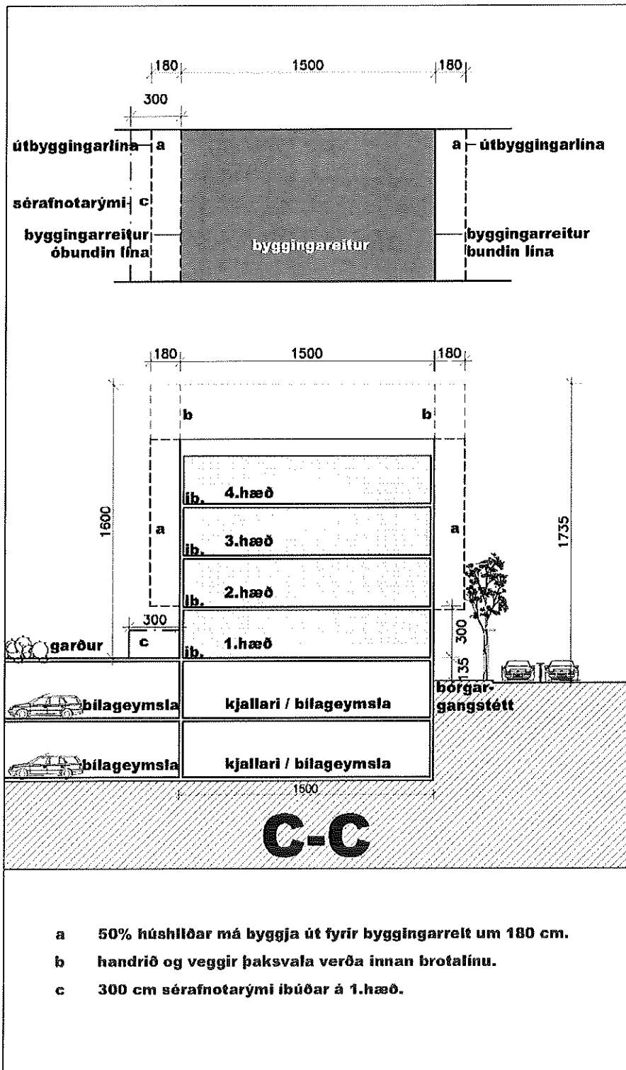
Skilmálasnið C-C
