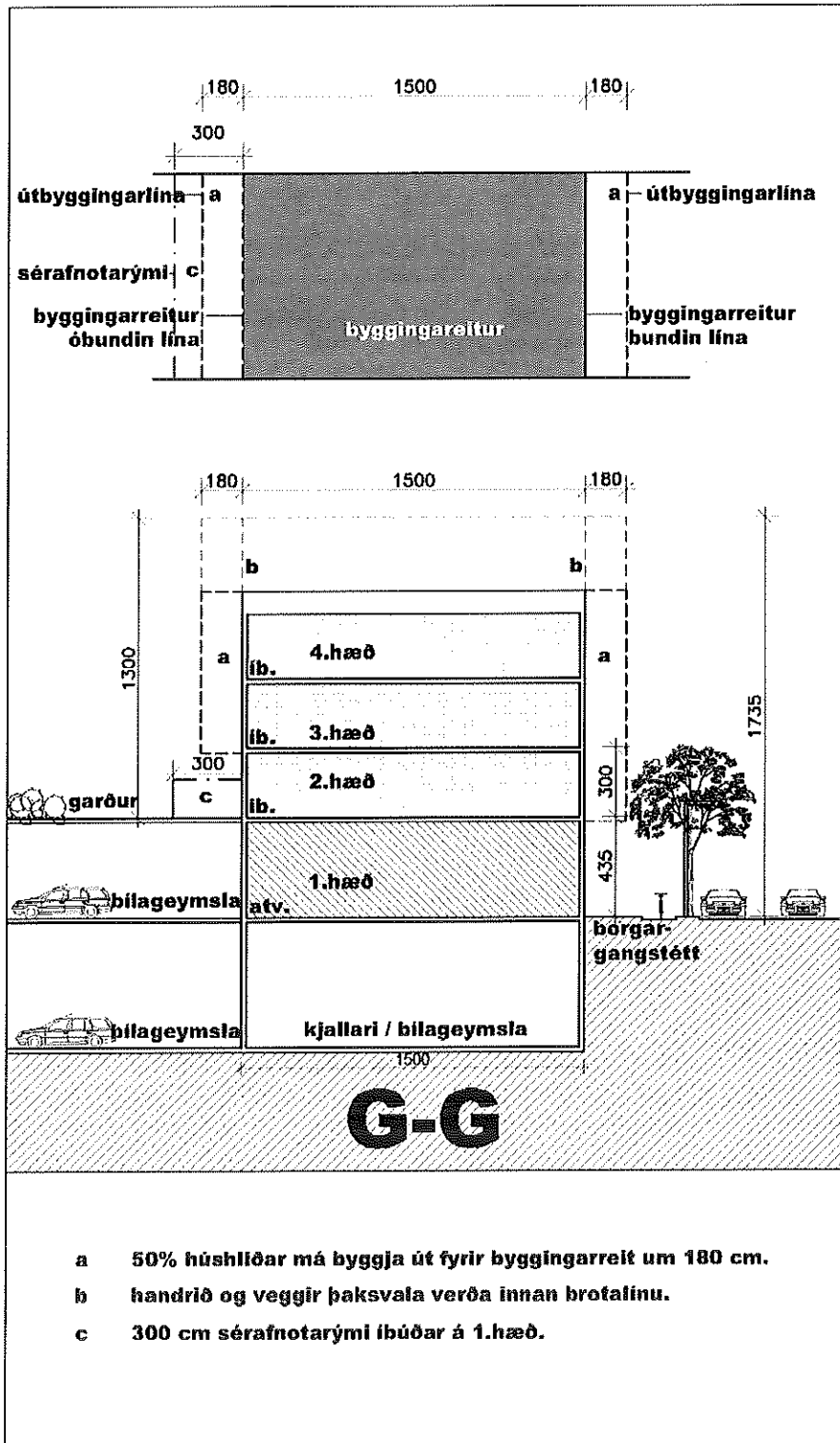
Skilmálasnið G-G
