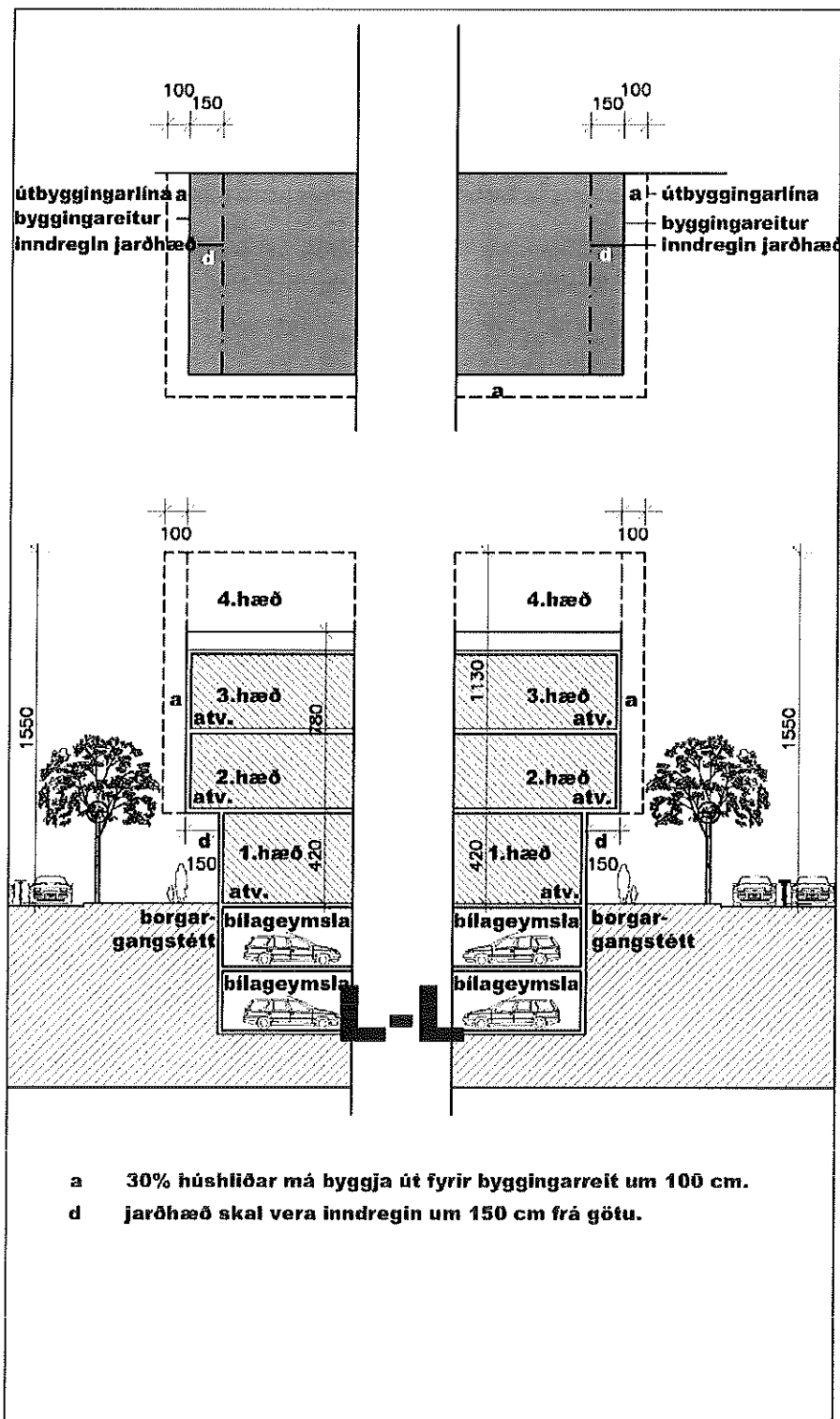
Skilmálasnið L-L
