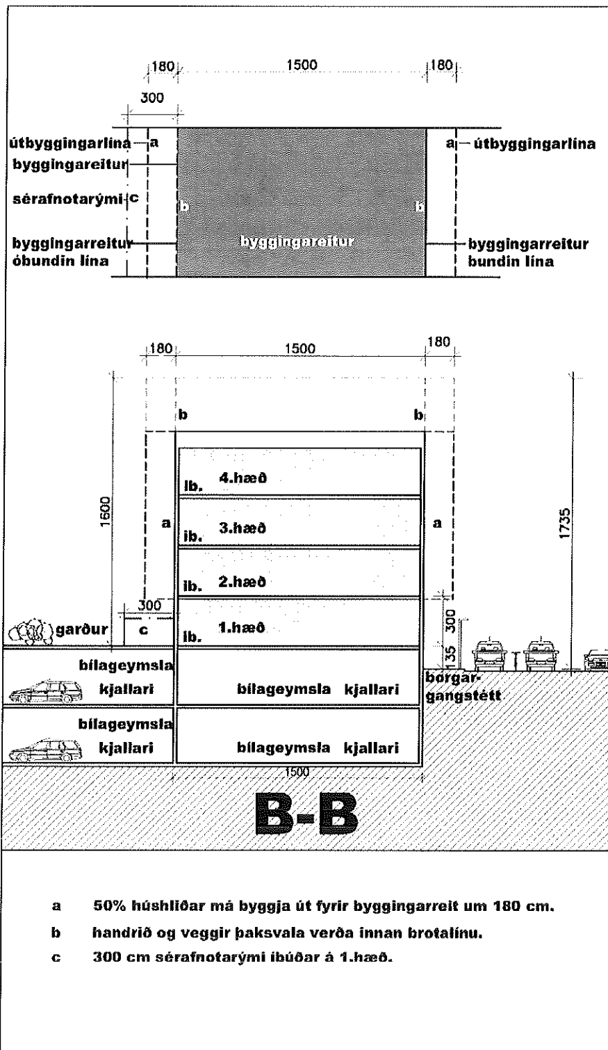
Skilmálasnið B-B
