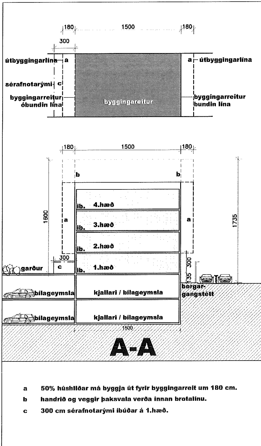
Skilmálasnið A-A
