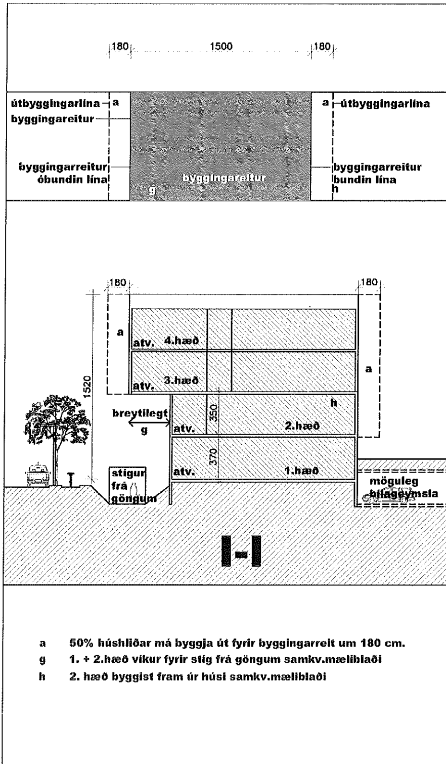
Skilmálasnið I-I
