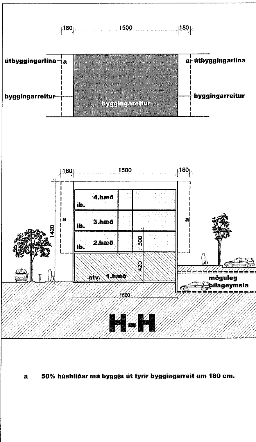
Skilmálasnið H-H
