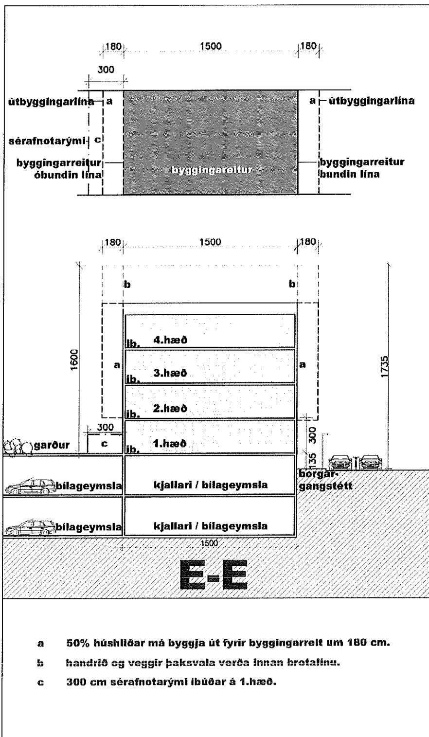
Skilmálasnið E-E
