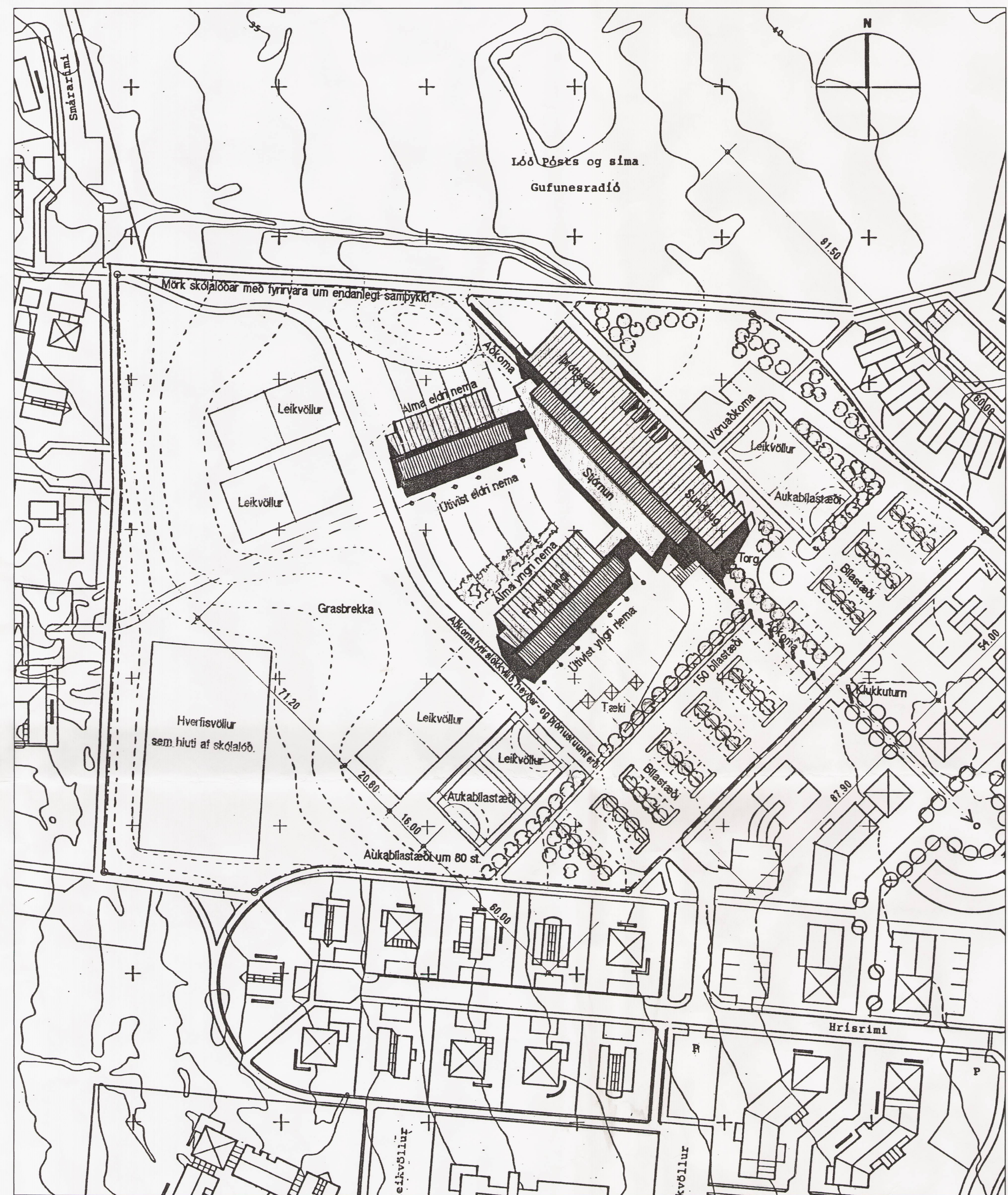
DEILISKIPULAG RIMASKÓLA SAMÞYKKT BORGRÁÐI 14.11.1992 M : 1/1000
