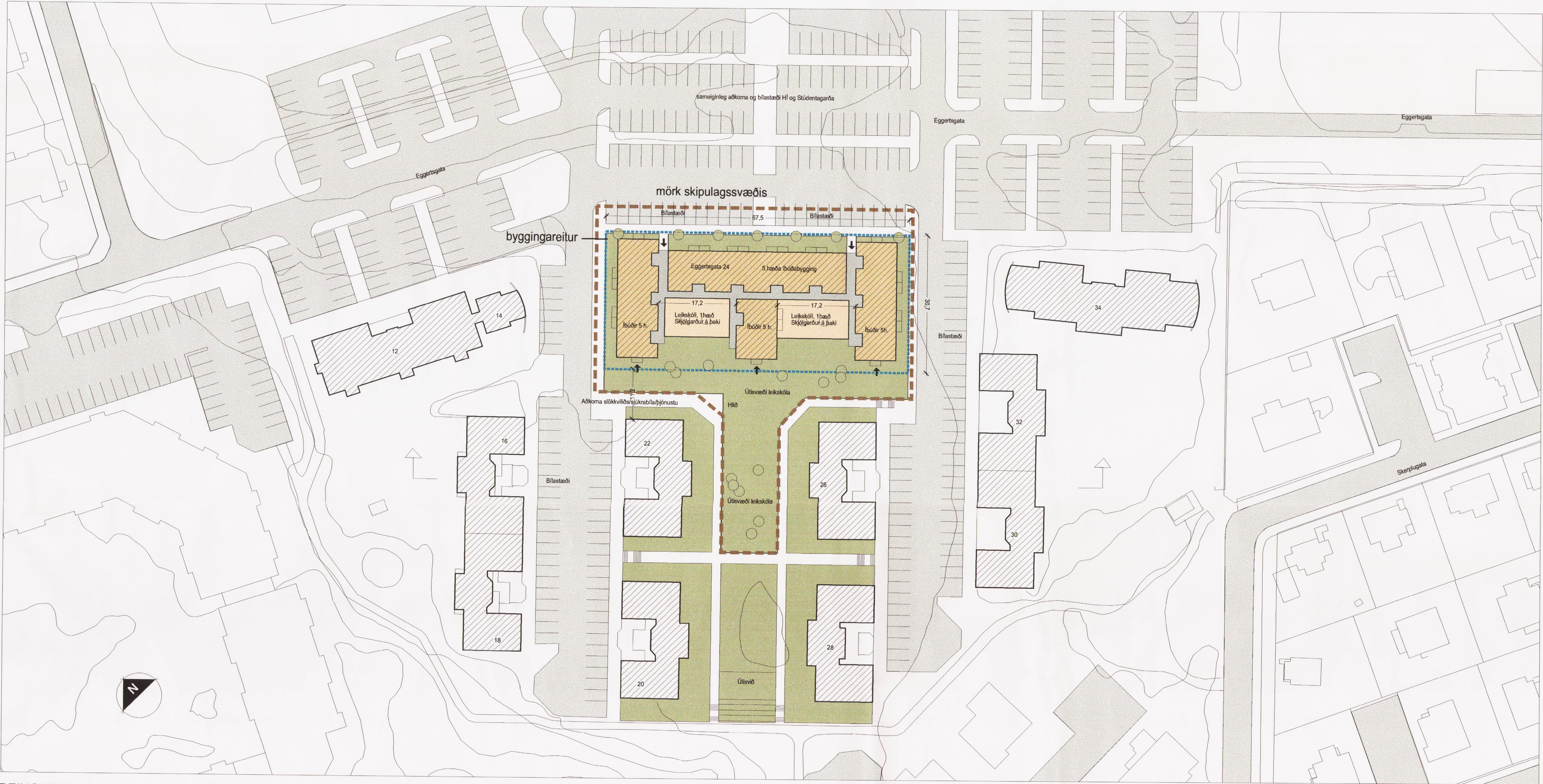
DEILISKIPULAG FYRIR EGGERTSGÖTU 24 M 1:500
