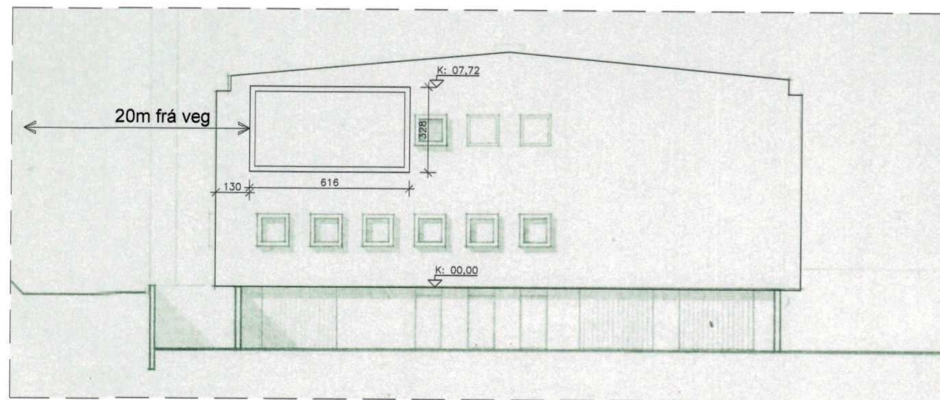
Útlit austurhlíð Sundaborg 1. 1:200
