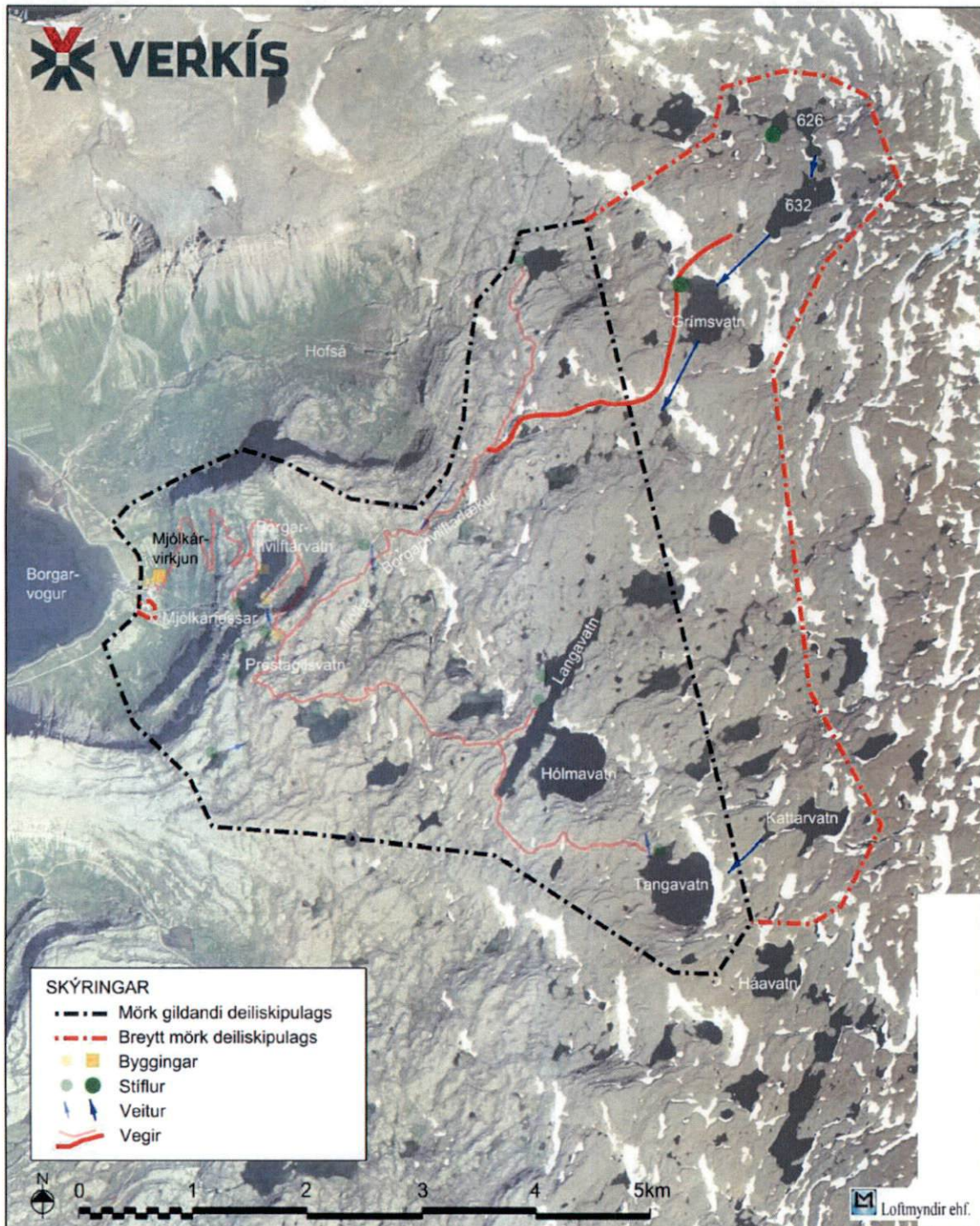
Mynd 3-1 Fyrirhugaðar framkvæmdir við Mjólkúrvirkjun. Núverandi mannvirki eru sýnd með daufum litum. Bláa örvarnar sýna fyrirhugaða vatnaflutninga en ekki nákvæma legu farvega.
