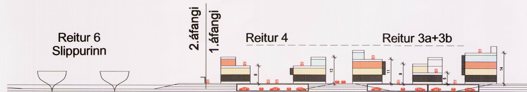
KENNISNIÐ AUSTUR-VESTUR 1:1000
