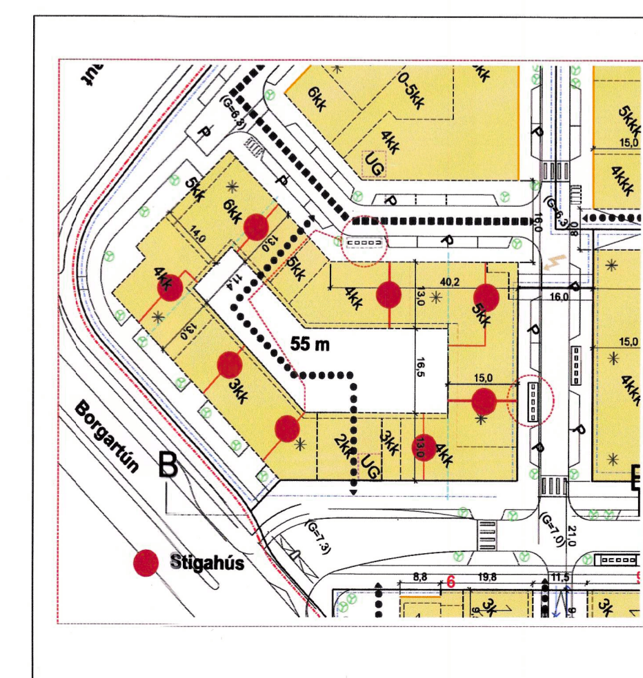
Staðsetning djúpgáma og hámarksfjarlægð frá stigahúsum.
