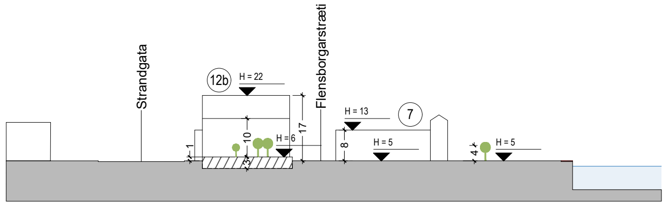
Sneiðing I-I
