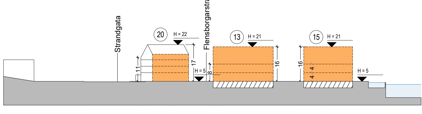
Sneiðing L-L
