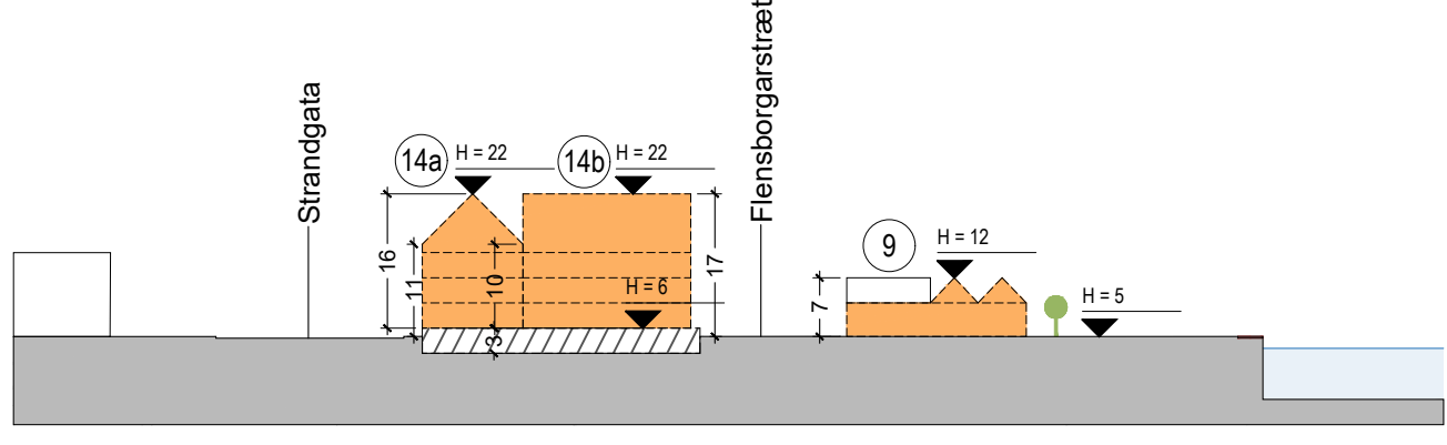
Sneiðing J-J
