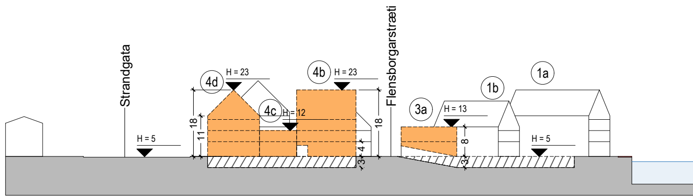
Sneiðing E-E
