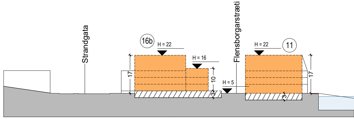
Sneiðing K-K
