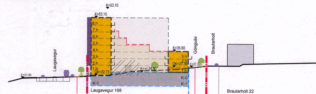
Sneiðing A-A
