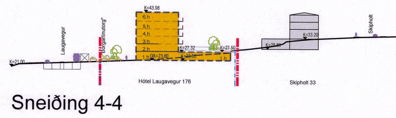
Sneiðing 4-4
