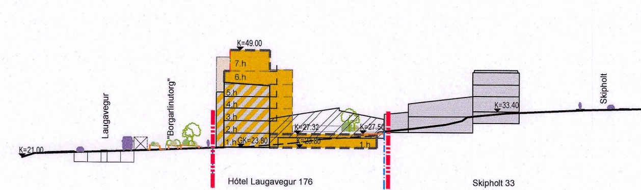
Sneiðing 3-3
