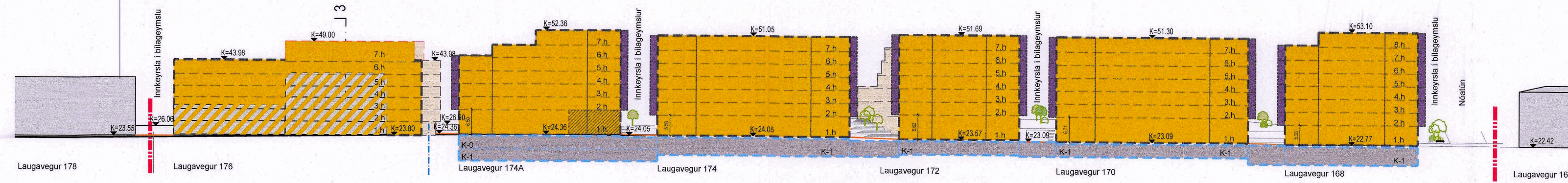
Sneiðing 1-1
