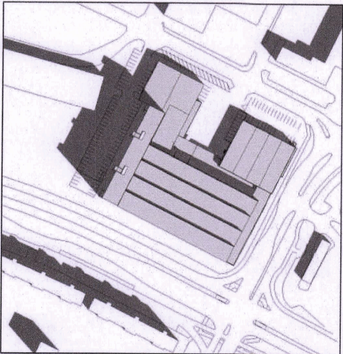
JAFNDÆGUR, 21 MARS 11:00
