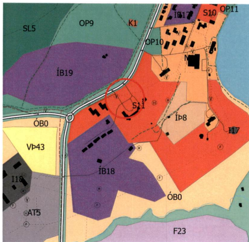
GILDANDI AÐALSKIPULAGSUPPDRÁTTUR
