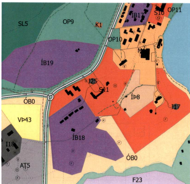
BREYTTUR AÐALSKIPULAGSUPPDRÁTTUR
