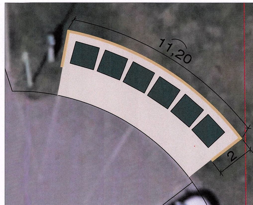
SKÝRINGARMYND MKV. 1:100
