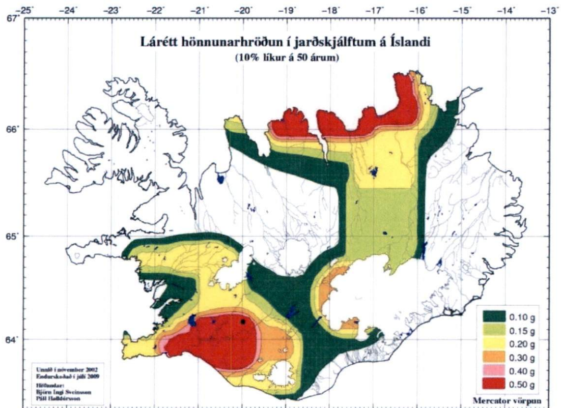
MYND 10. Kort af Íslandi sem sýnir lárétta grunnhröðun fyrir stöðugleikagreiningu mannvirkja. Sveitarfélagið liggur að mestu innan hæsta áhættuflokks með hönnunarhröðun 0,5*g 26 .
