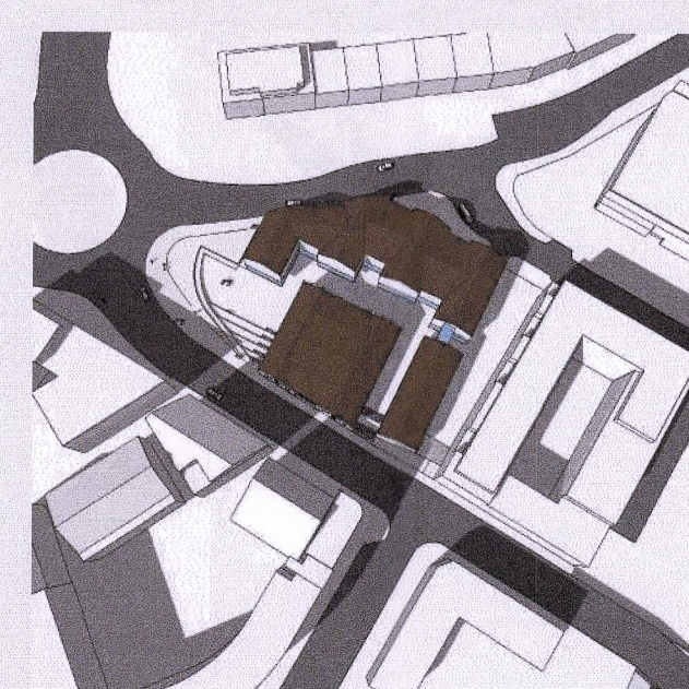
21.6 SUMARSÓLSTÖÐUR // KL. 16.00
