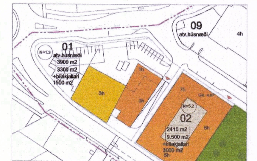
DEILISKIPULAG SAMÞ. 2013
