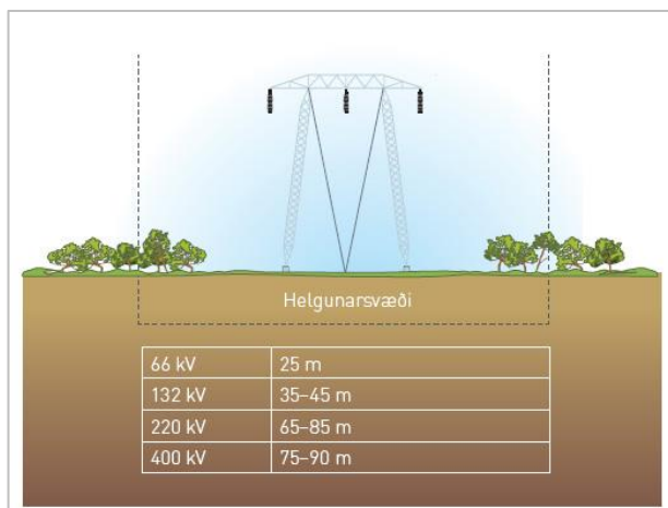
MYND 2. Helgunarsvæði háspennulína skv. staðli ÍST EN 50341-3-12:2001.
