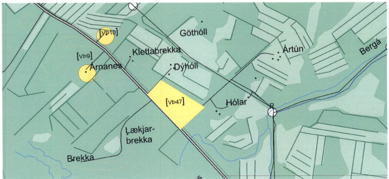
BREYTTUR AÐALSKIPULAGSUPPDRAÐTUR 1:15.000
