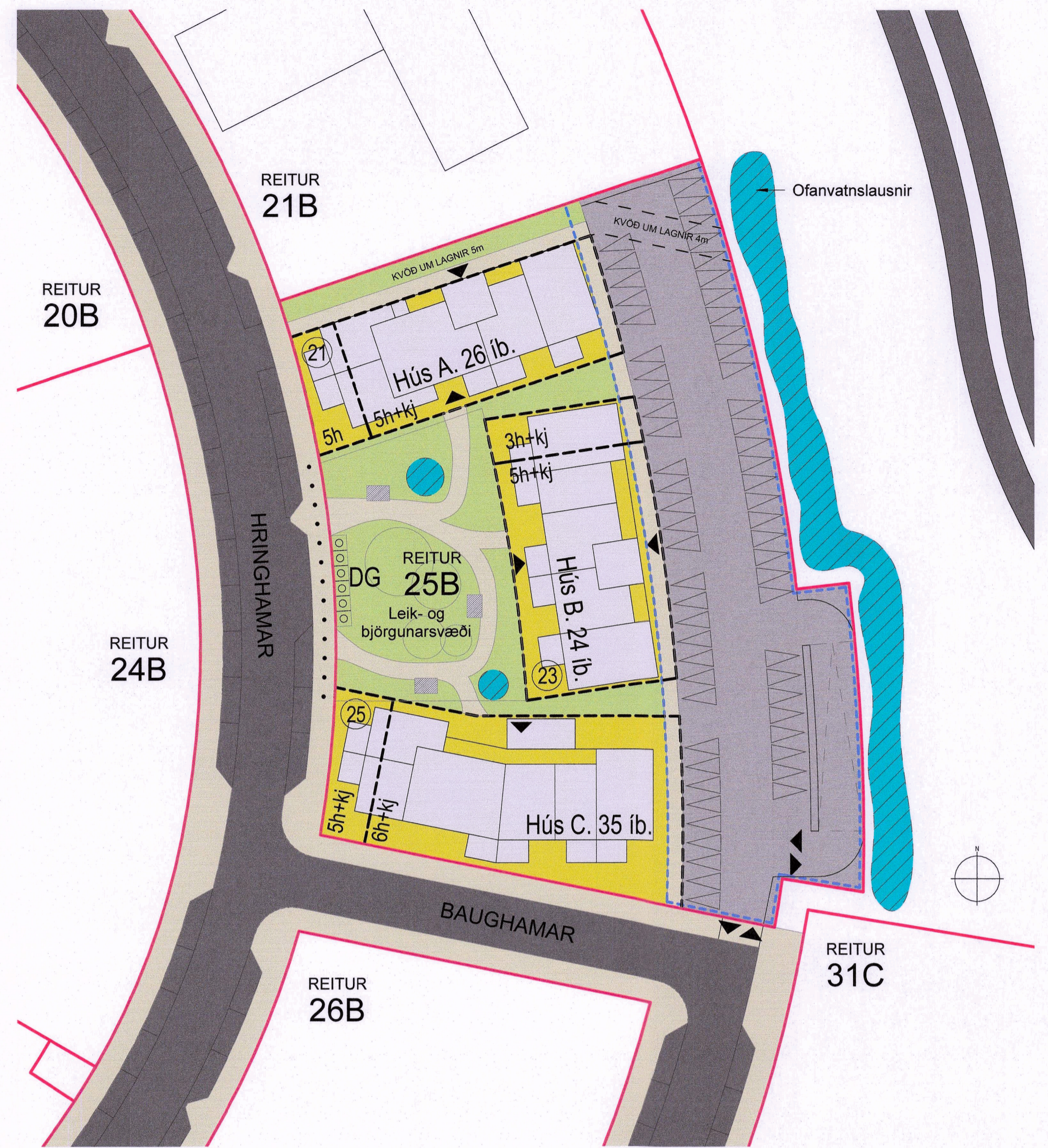
Skýringarmynd 1:500
