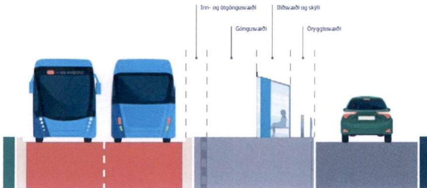
Mynd 6 Þversnið af brautarpalli fyrir Borgarlínu. Heimild: Borgarlínan 1. lota frumdrög.
