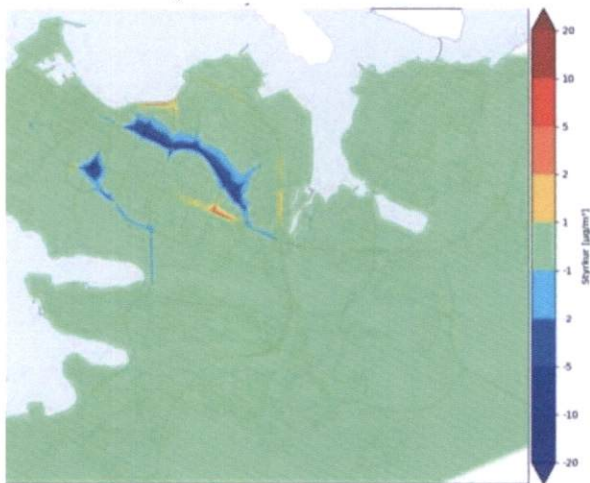
Mynd 9 Breyting á ársmeðalstyrk \text{PM}_{10} með Borgarlínu, miðað við núllkost.
