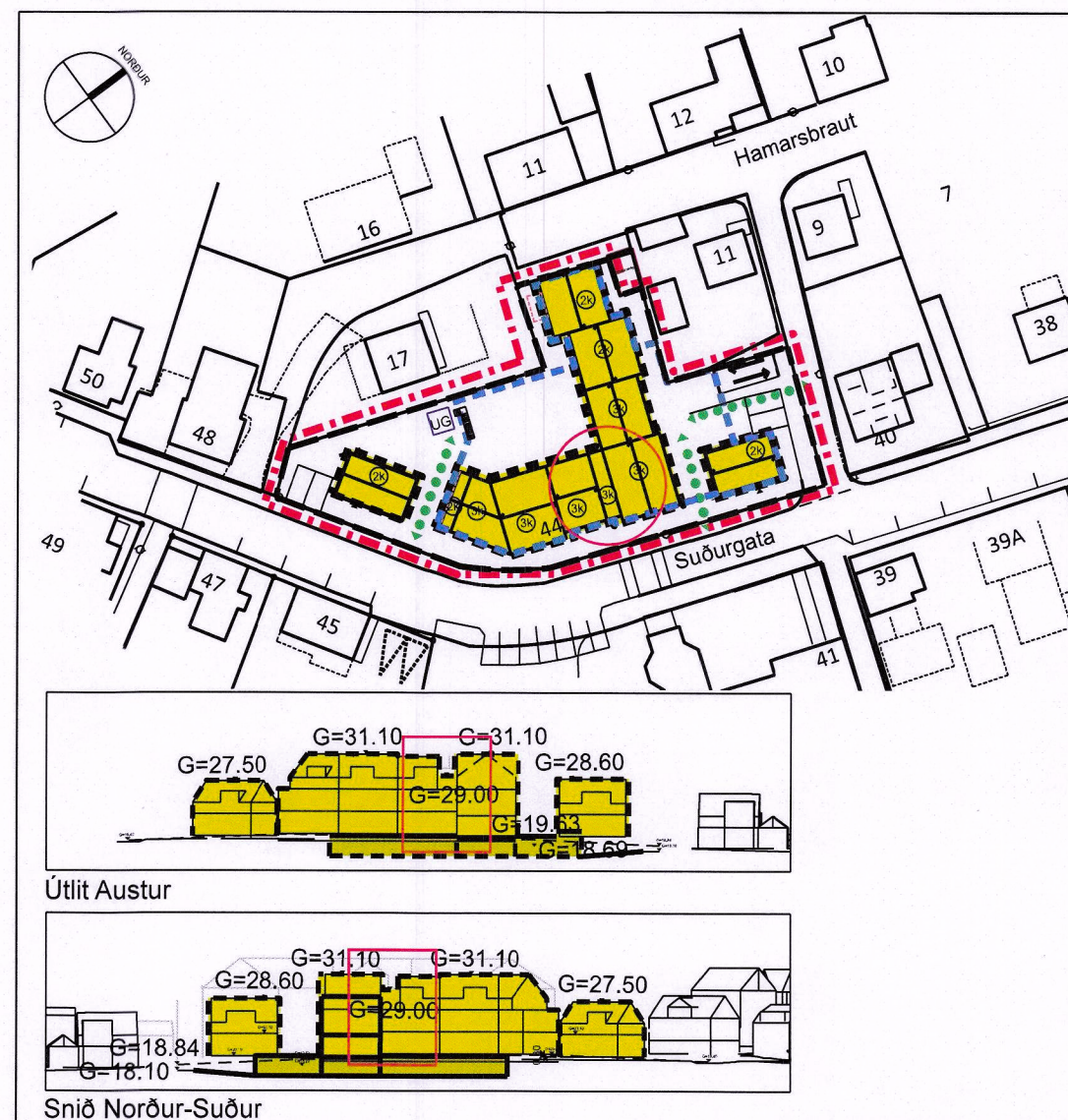
EFTIR BREYTINGU 1:1000
