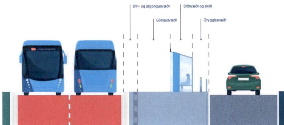
Mynd 4.1 Dæmi um þversnið af brautarpalli fyrir Borgarlínu. Heimild: Borgarlínan 1. lota Frumdrög .
