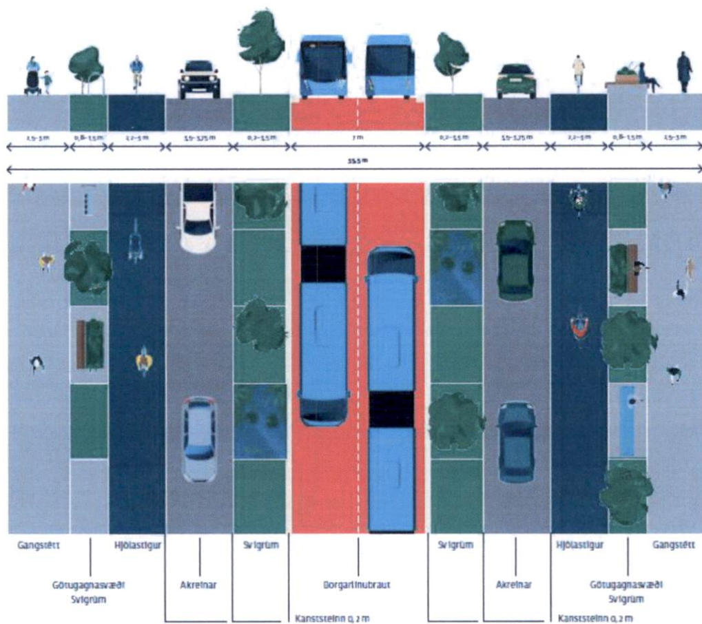
Mynd 4.2 Snið Borgarlínuötu sem sýnir æskilegar götueiningar og samspil þeirra. Heimild: Borgarlínan 1. Iota Frumdrög .
