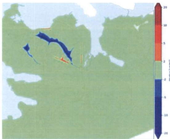
Mynd 7 Breyting á ársmeðalstyrk \text{NO}_2 með Borgarlínu. Blár litur þýðir minni loftmengun að ársmeðaltali, rauður meiri mengun.
