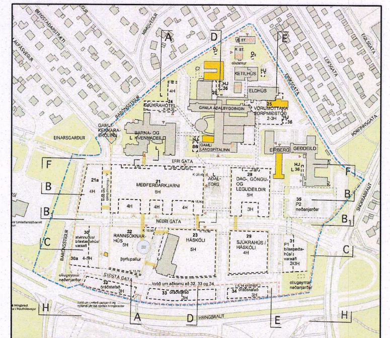
DEILISKIPULAG LANSPÍTALANS VIÐ HRINGBRAUT Staðfest í B deild Stjórnartíðinda 8. apríl 2013
