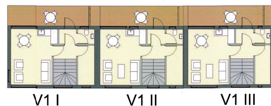
Veghúsastígur 1 - 1.hæð 1 : 200
