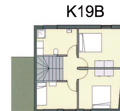
Klapparstígur 19 - Rishæð 1 : 200
