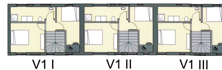
Veghúsastígur 1 - Rishæð 1 : 200
